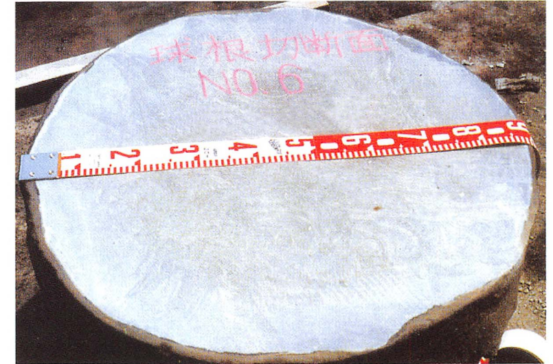
拡大球根の性状は、砂層地盤の場合の例では完全なモルタル状の密な硬化体となっております。(コア圧縮強度については、その一例として8ページに示しております。)
