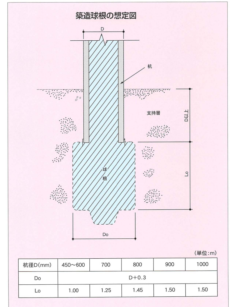
拡大球根の性状は、砂層地盤の場合の例では完全なモルタル状の密な硬化体となっております。(コア圧縮強度については、その一例として8ページに示しております。)
